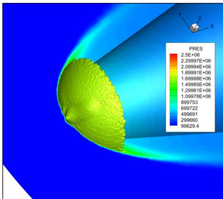
Рисунок 4.49 – Результат численного моделирования распределения ударной волны для затупленного конуса при M = 10 с использованием расчетных кодов UST3D
