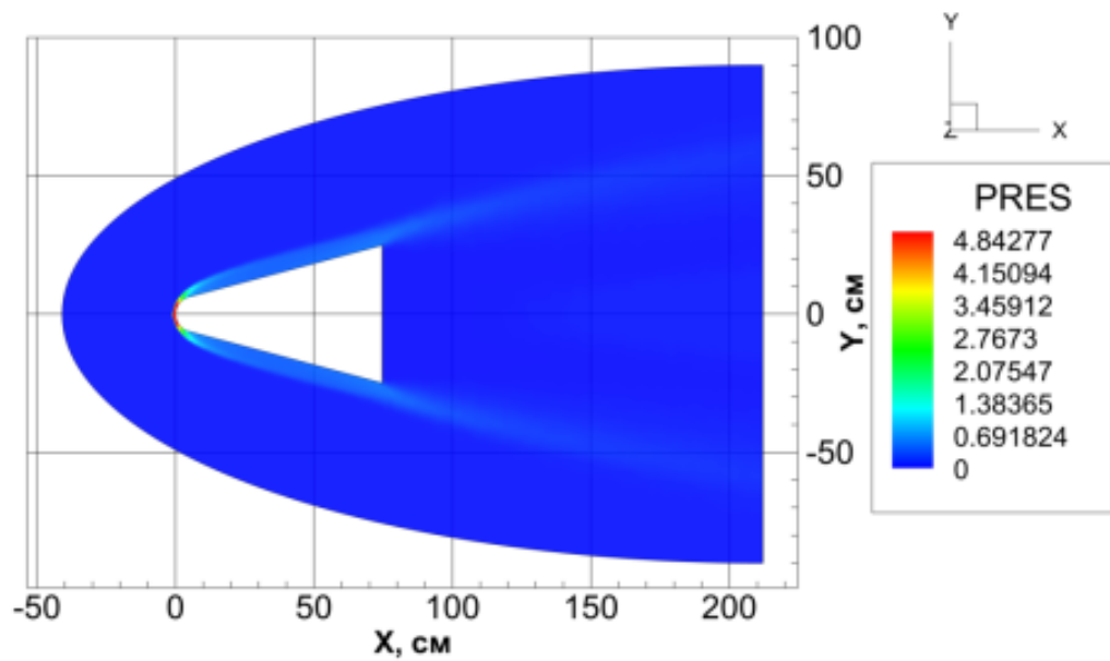
Рисунок 4.53 – Распределение давления на пространственной неструктурированной тетраэдральной расчетной сетке при M = 10 в результате работы компьютерного кода UST3D_AUSM_UP2
