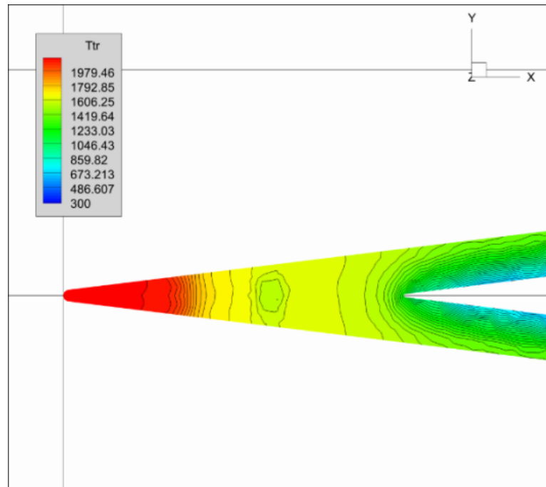
Рисунок 4.95 – Распределение температуры в области составной носовой части экспериментального летательного аппарата NIFiRE-1 без юбки
