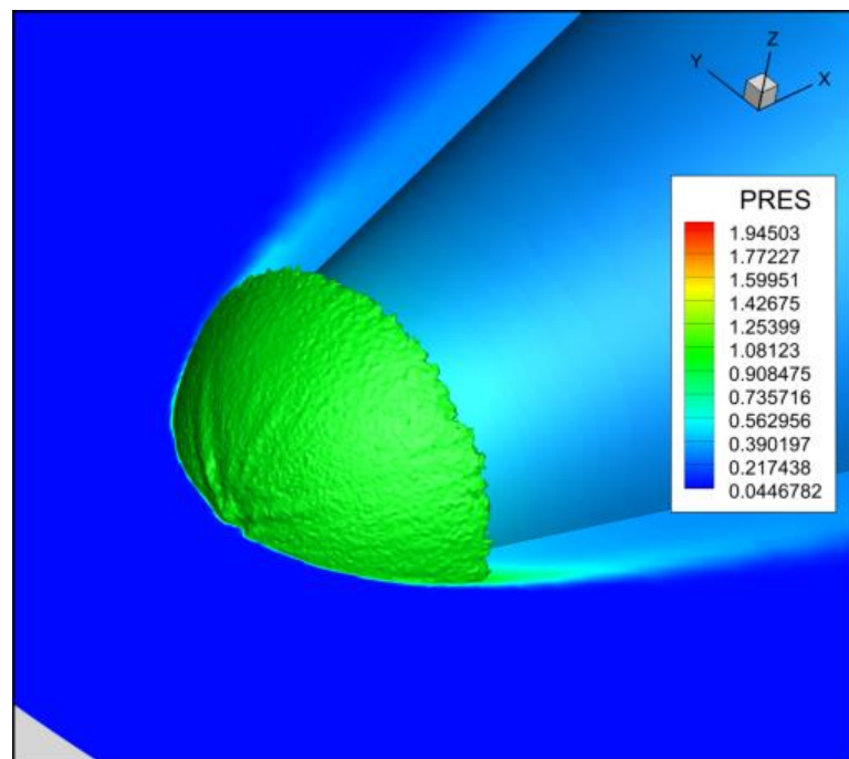
Рисунок 4.46 – Результат численного моделирования распределения ударной волны для затупленного конуса при M = 13 с использованием расчетных кодов UST3D_AUSMUP2
