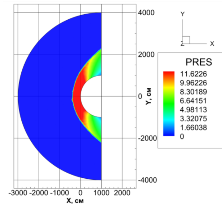
Рисунок 4.39 – Распределение давления на 8-ми млн пространственной неструктурированной тетраэдральной расчетной сетке в результате работы компьютерного кода UST3D_AUSMPW
