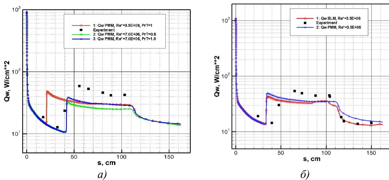
Рисунок 4.81 – Графики плотности конвективных тепловых потоков вдоль поверхности [199], которые использовались при расчетах
