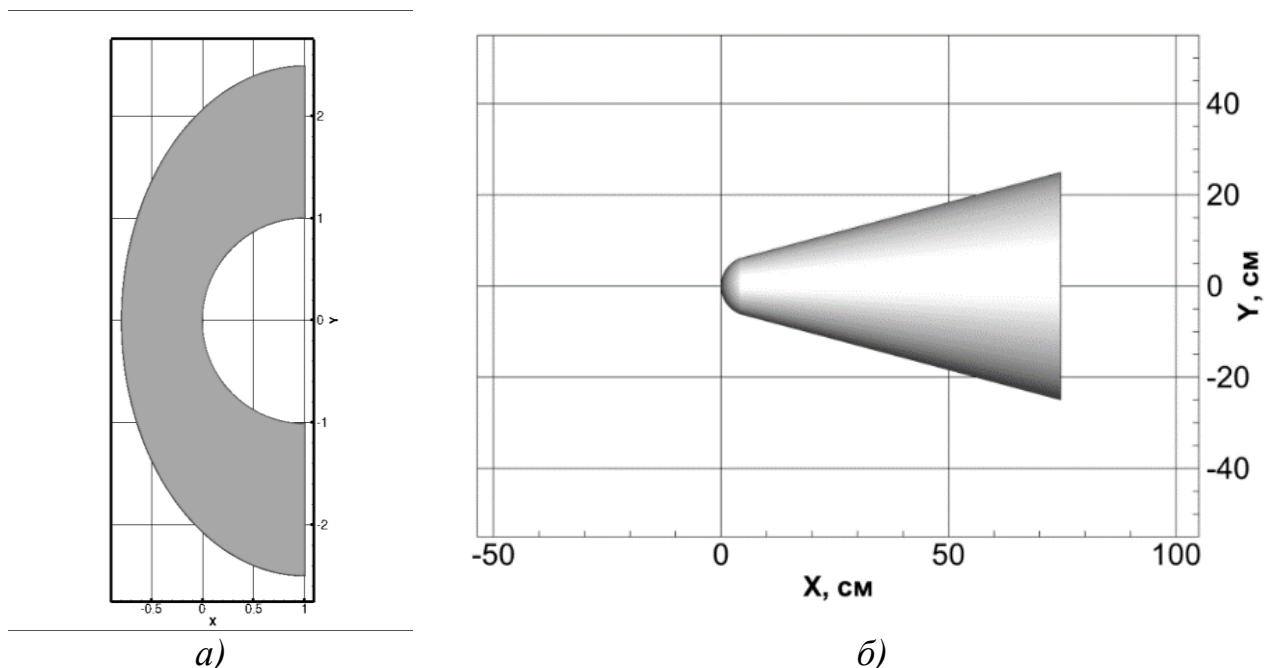
Рисунок 4.20 – Виртуальные геометрические модели. а) модель бесконечного цилиндра; б) модель конуса, затупленного по сфере
