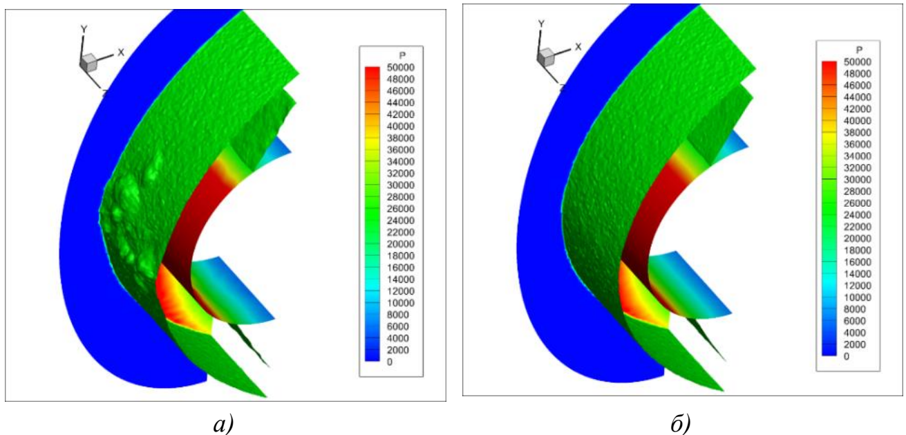
Рисунок 4.23 – Результаты численного моделирования распределения ударной волны для бесконечного цилиндра с использованием расчетного кода: а) HySol точным методом; б) HySol методом AUSM \pm up
