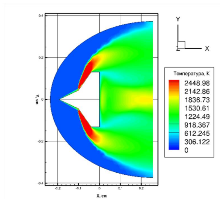
Рисунок 4.15 – Распределение температуры в результате работы компьютерного кода HySol
