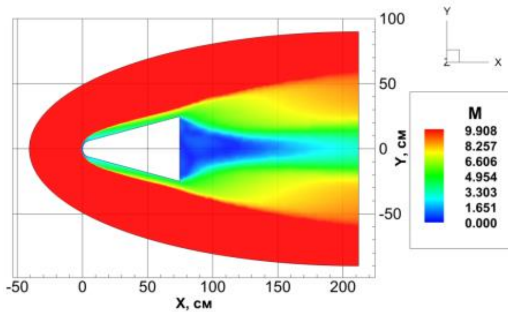
Рисунок 4.57 – Распределение чисел Маха на пространственной неструктурированной тетраэдральной расчетной сетке при M = 13 в результате работы компьютерного кода UST3D_AUSM_UP2
