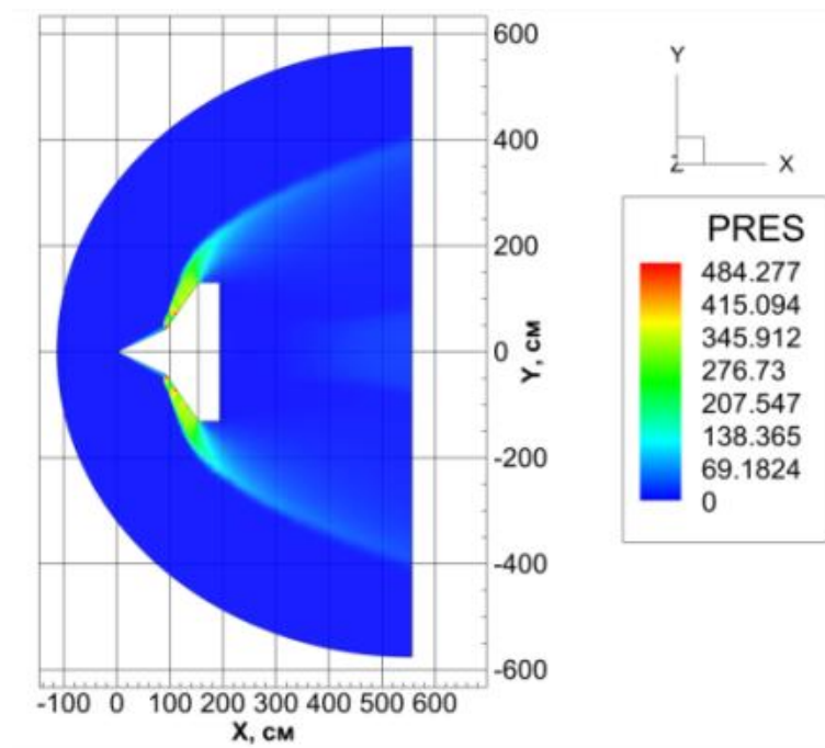
Рисунок 4.10 – Распределение давления в результате работы компьютерного кода UST3D_AUSM_UP2
