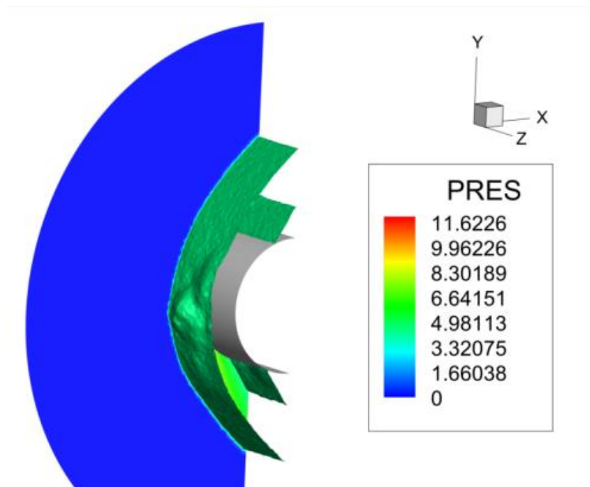
Рисунок 4.26 – Результаты численного моделирования распределения ударной волны для бесконечного цилиндра с использованием расчетного кода UST3D
