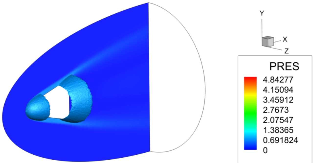
Рисунок 4.45 – Результат численного моделирования распределения ударной волны для затупленного конуса при M = 13 с использованием расчетного кода UST3D_AUSMUP2
