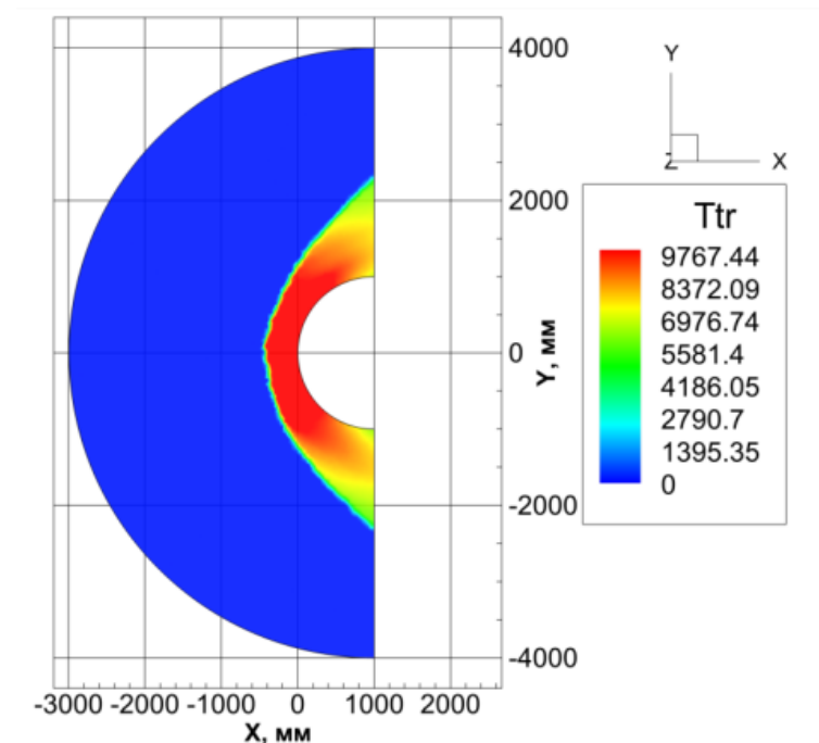
Рисунок 4.33 – Распределение температуры на 2-х млн пространственной неструктурированной тетраэдральной расчетной сетке в результате работы компьютерного кода UST3D_AUSM_UP2
