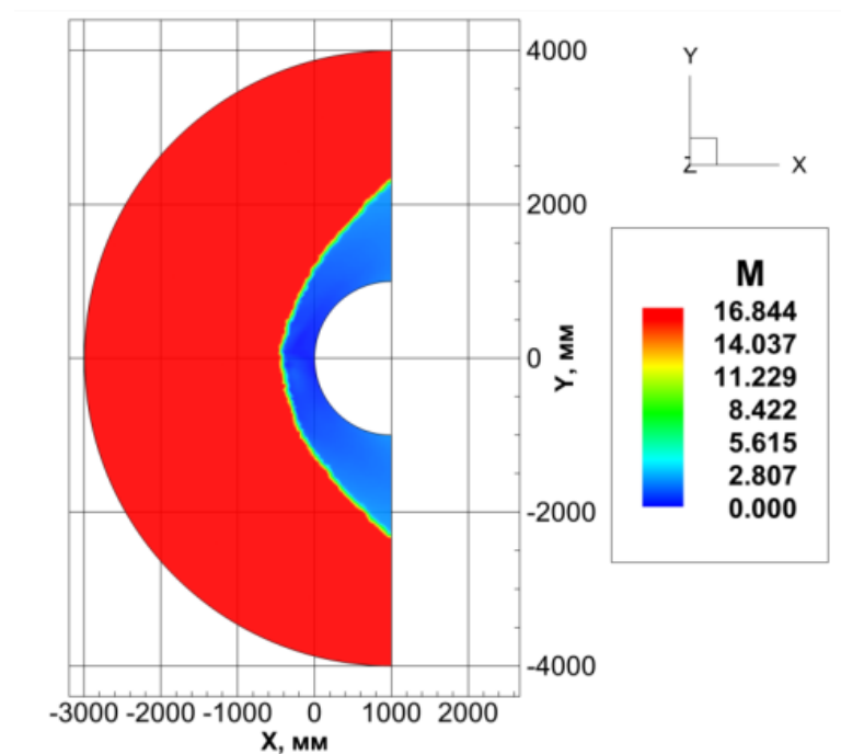
Рисунок 4.27 – Распределение чисел Маха на 2-х млн пространственной неструктурированной тетраэдральной расчетной сетке в результате работы компьютерного кода UST3D_AUSM_UP2
