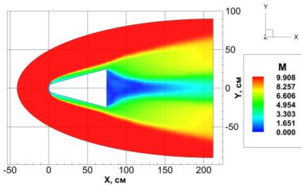
Рисунок 4.51 – Распределение чисел Маха на пространственной неструктурированной тетраэдральной расчетной сетке при M = 10 в результате работы компьютерного кода UST3D_AUSM_UP2
