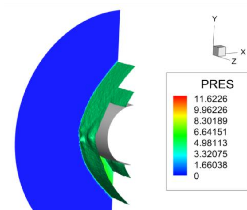
Рисунок 4.25 – Результаты численного моделирования распределения ударной волны для бесконечного цилиндра с использованием расчетного кода UST3D_AUSMUP2
