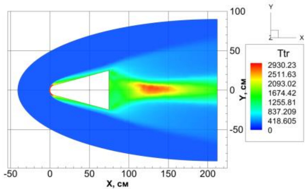
Рисунок 4.55 – Распределение температуры на пространственной неструктурированной тетраэдральной расчетной сетке при M = 10 в результате работы компьютерного кода UST3D_AUSM_UP2
