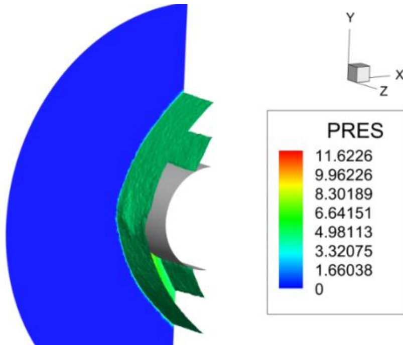
Рисунок 4.24 – Результаты численного моделирования распределения ударной волны для бесконечного цилиндра с использованием расчетного кода UST3D_AUSMPW
