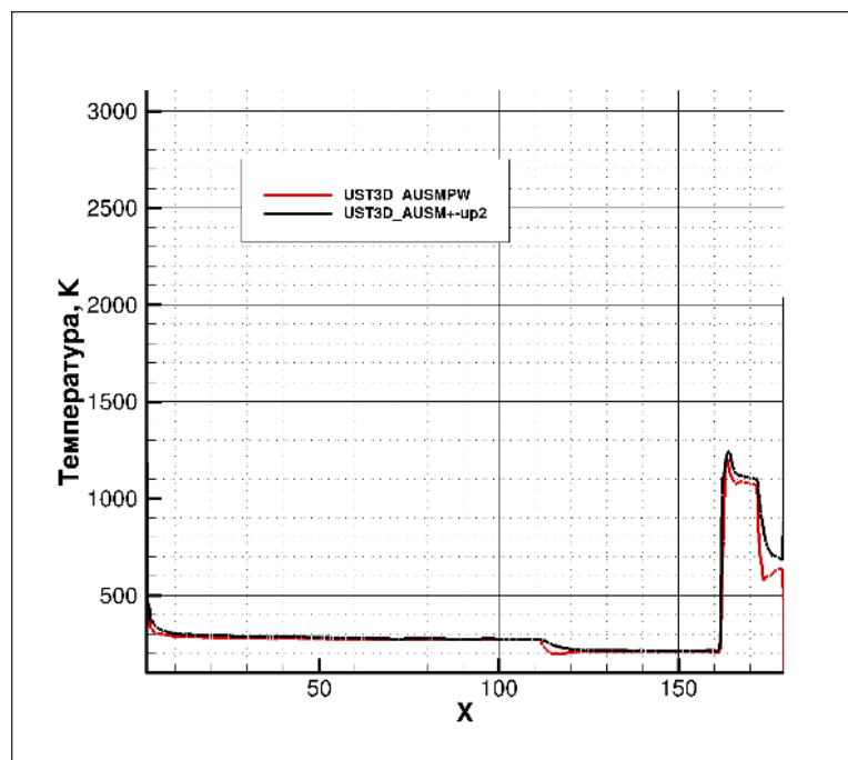
Рисунок 4.70 – Сравнение результатов полученных с помощью разработанного компьютерного кода с результатами компьютерного кода UST3D_AUSMPW [*] для температуры при нулевом угле атаки
