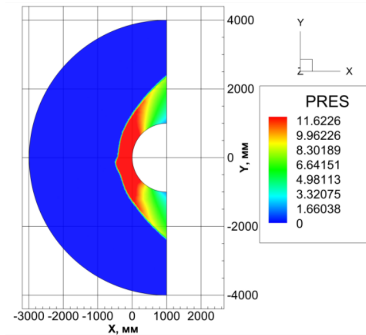
Рисунок 4.38 – Распределение давления на 8-ми млн пространственной неструктурированной тетраэдральной расчетной сетке в результате работы компьютерного кода UST3D_AUSM_UP2
