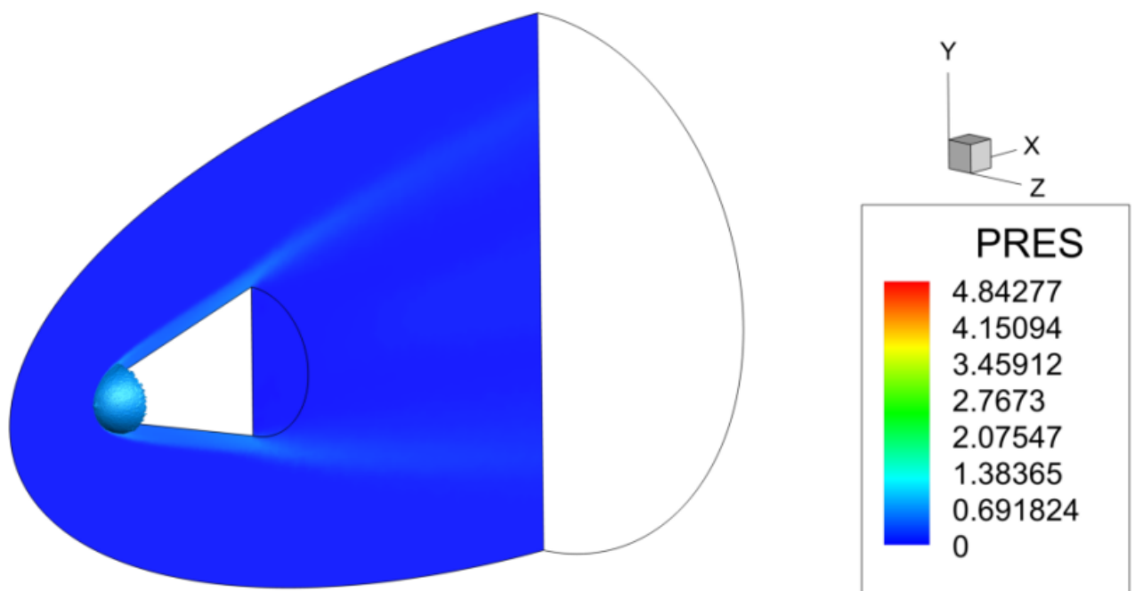
Рисунок 4.42 – Результат численного моделирования распределения ударной волны для затупленного конуса при M = 10 с использованием расчетного кода
