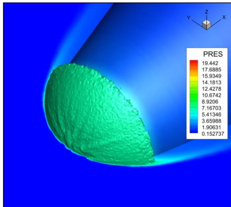
Рисунок 4.48 – Результат численного моделирования распределения ударной волны для затупленного конуса при M = 10 с использованием расчетных кодов UST3D_AUSMUP2
