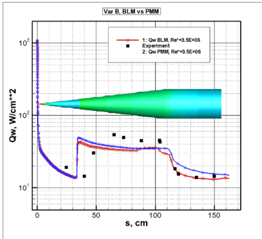
Рисунок 4.83 – Распределение конвективных тепловых потоков вдоль поверхности летательного аппарата, использованных при расчете теплового баланса оболочки
