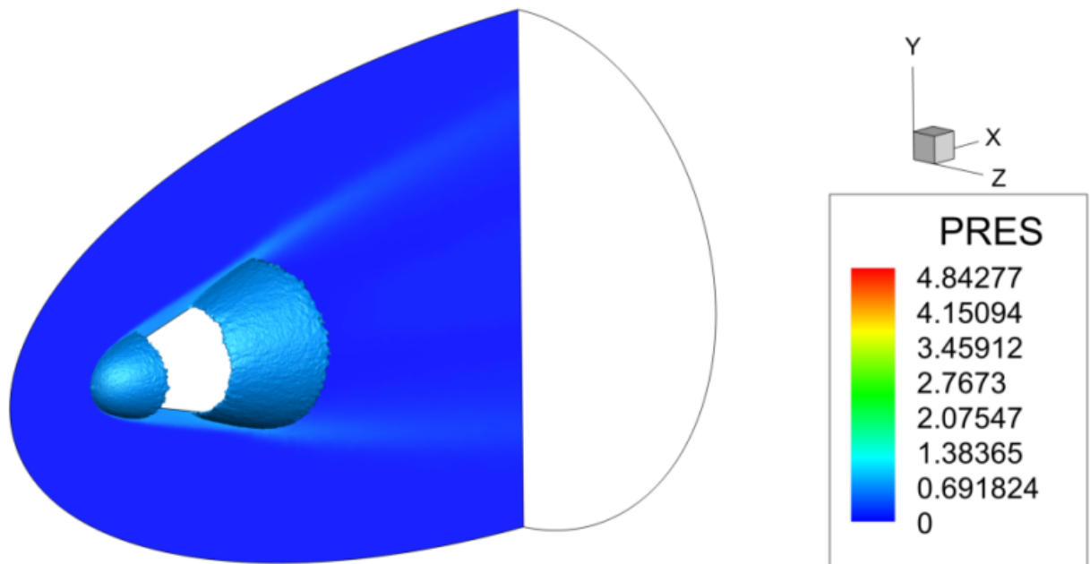
Рисунок 4.44 – Результат численного моделирования распределения ударной волны для затупленного конуса при M = 13 с использованием расчетного кода UST3D_AUSMPW
