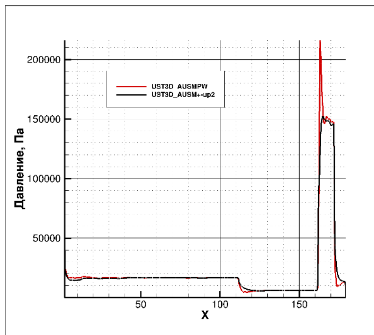
Рисунок 4.68 – Сравнение результатов полученных с помощью разработанного компьютерного кода с результатами компьютерного кода UST3D_AUSMPW [*] для давления при нулевом угле атаки
