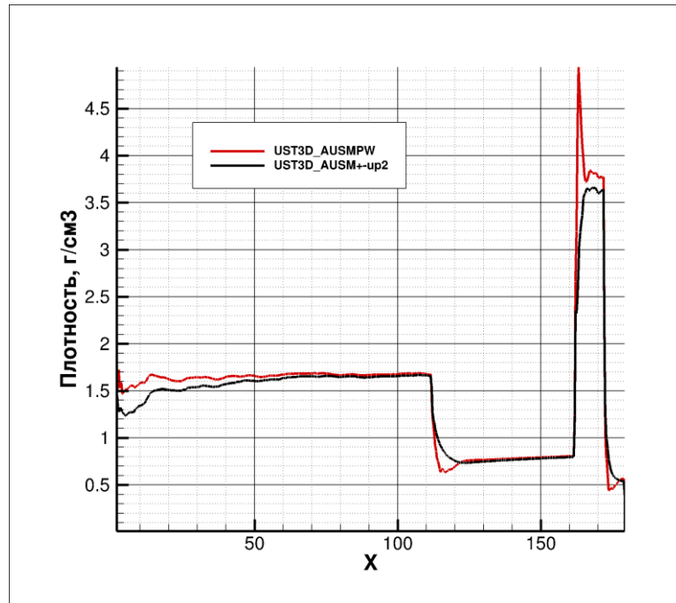
Рисунок 4.69 – Сравнение результатов полученных с помощью разработанного компьютерного кода с результатами компьютерного кода UST3D_AUSMPW [*] для плотности при нулевом угле атаки
