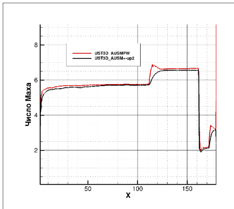
Рисунок 4.67 – Сравнение результатов полученных с помощью разработанного компьютерного кода с результатами компьютерного кода UST3D_AUSMPW [*] для числа Маха при нулевом угле атаки
