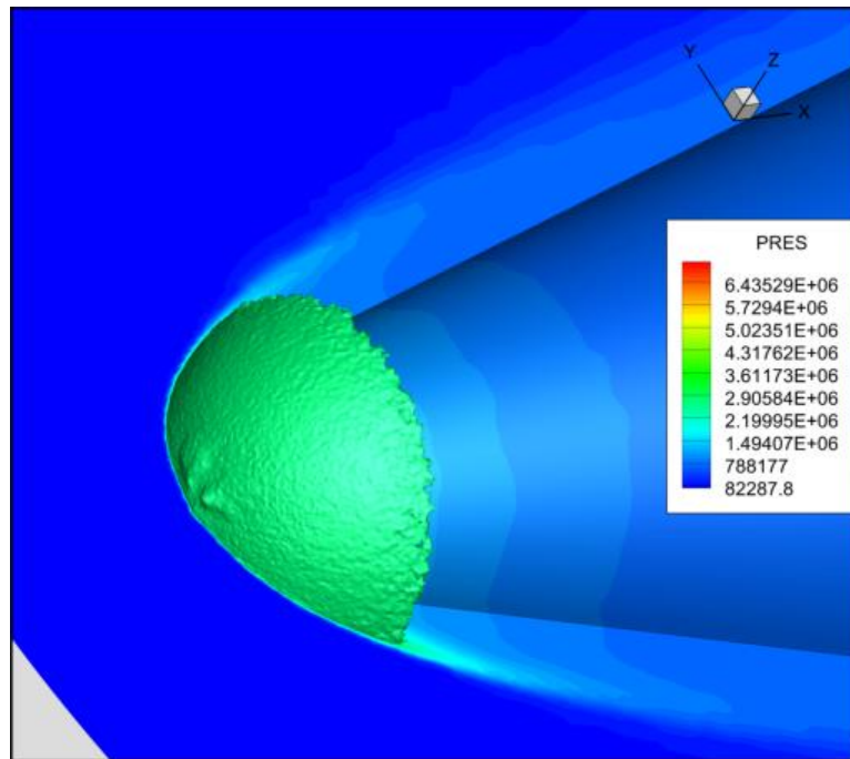
Рисунок 4.47 – Результат численного моделирования распределения ударной волны для затупленного конуса при M = 13 с использованием расчетных кодов UST3D
