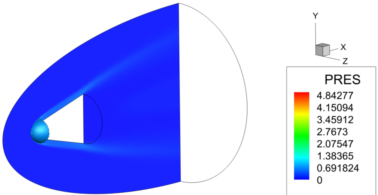
Рисунок 4.43 – Результат численного моделирования распределения ударной волны для затупленного конуса при M = 10 с использованием расчетного кода UST3D_AUSMUP2
