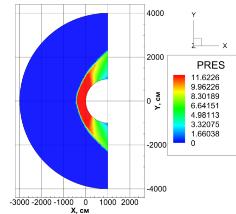
Рисунок 4.31 – Распределение давления на 2-х млн пространственной неструктурированной тетраэдральной расчетной сетке в результате работы компьютерного кода UST3D_AUSMPW
