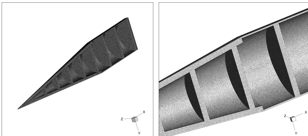
Рисунок 4.85 – Неструктурированная тетраэдральная сетка, с равномерным распределением ячеек по всей расчетной области
