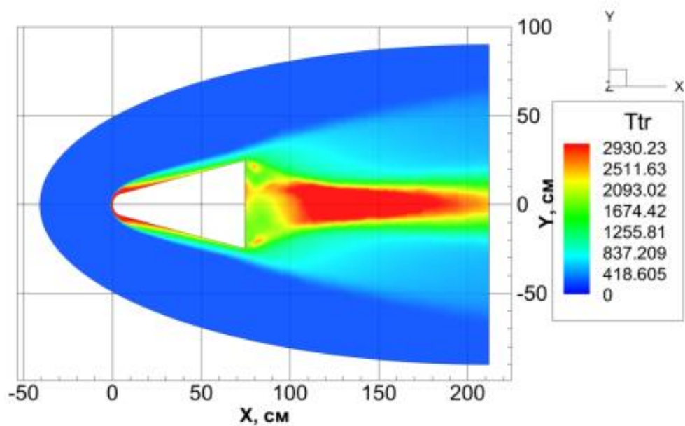
Рисунок 4.61 – Распределение температуры на пространственной неструктурированной тетраэдральной расчетной сетке при M = 13 в результате работы компьютерного кода UST3D_AUSM_UP2
