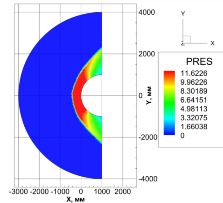
Рисунок 4.30 – Распределение давления на 2-х млн пространственной неструктурированной тетраэдральной расчетной сетке в результате работы компьютерного кода UST3D_AUSM_UP2
