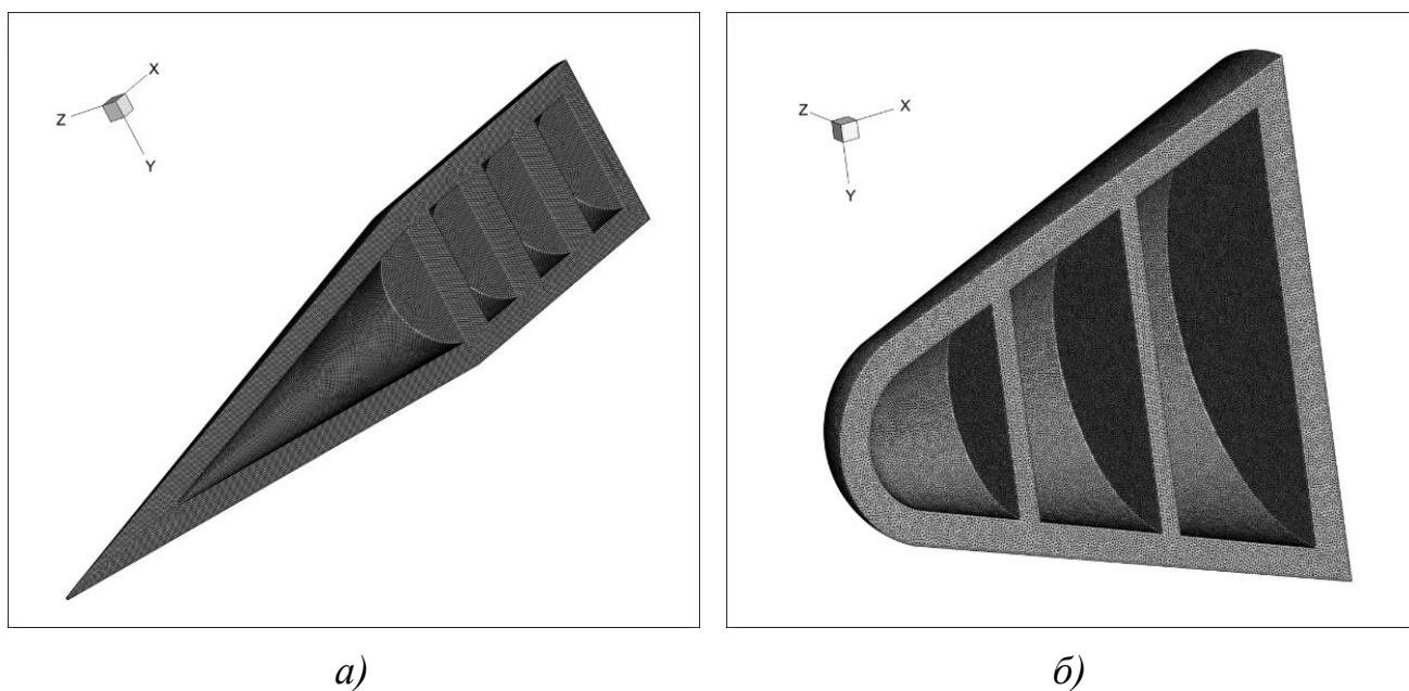
Рисунок 4.84 – Неструктурированная тетраэдральная сетка, с равномерным распределением ячеек по всей расчетной области: а) для экспериментального летательного аппарата NIFiRE-1; б) для конуса затупленного по сфере
