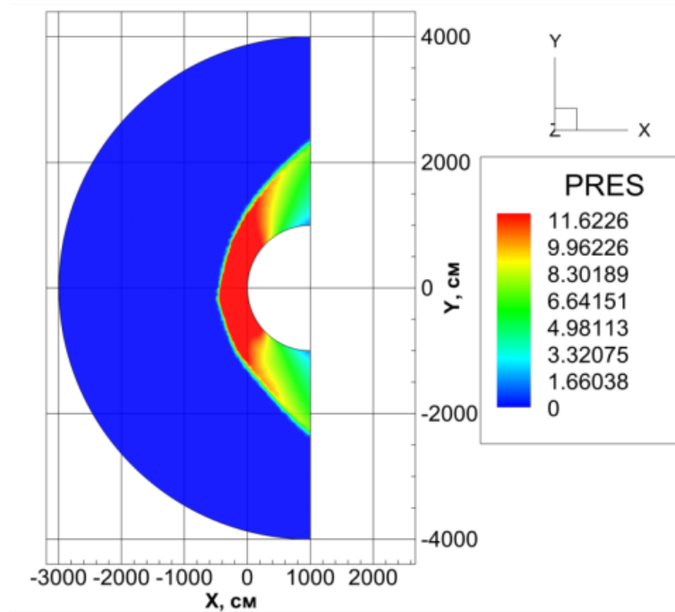
Рисунок 4.32 – Распределение давления на 2-х млн пространственной неструктурированной тетраэдральной расчетной сетке в результате работы компьютерного кода UST3D
