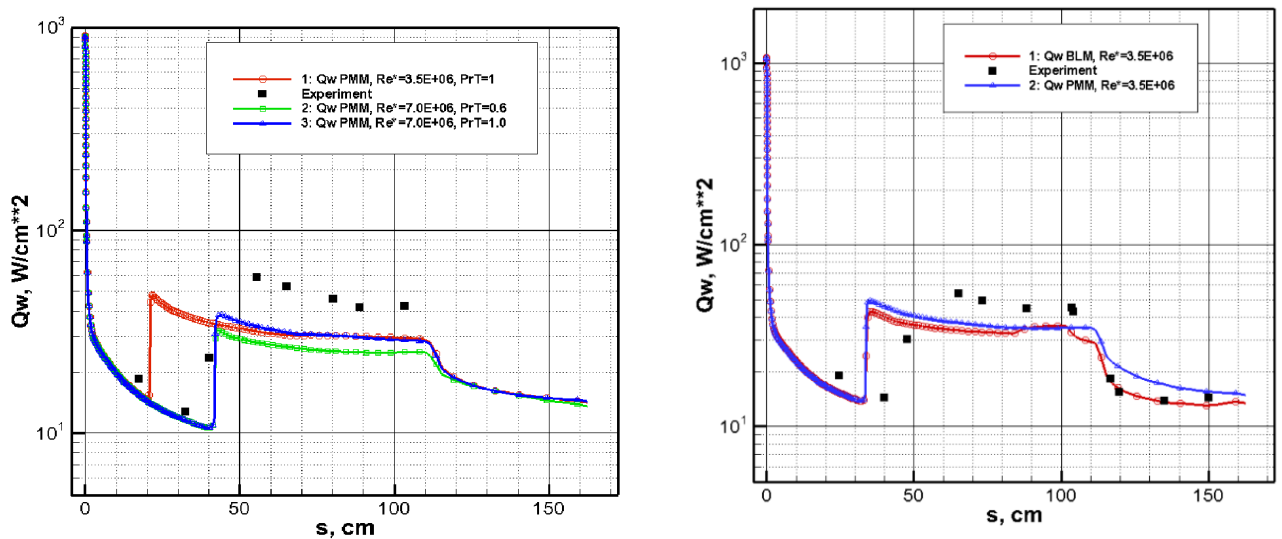
Рисунок 4.78 – Графики плотности конвективных тепловых потоков вдоль поверхности [1], которые использовались при расчетах.
