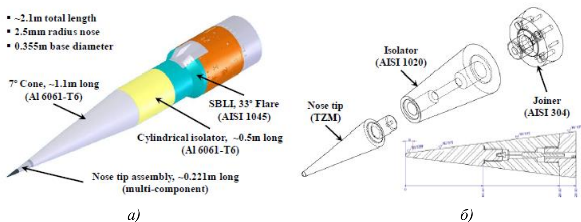
Рисунок 4.79 – Схема исследовательского летательного аппарата HIFiRE-1 [202].
