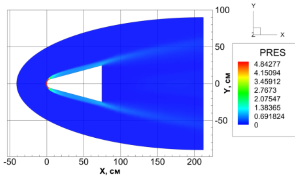
Рисунок 4.59 – Распределение давления на пространственной неструктурированной тетраэдральной расчетной сетке при M = 13 в результате работы компьютерного кода UST3D_AUSM_UP2
