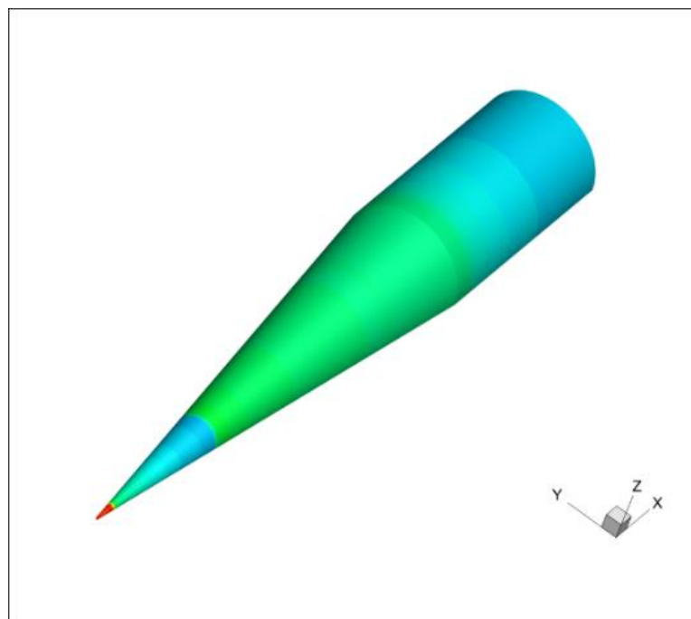
Рисунок 4.82 – Экстраполяция двухмерного распределения конвективных тепловых потоков вдоль поверхности летательного аппарата на его трехмерную модель
