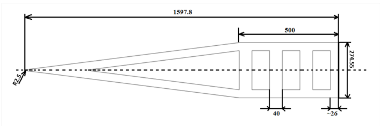
Рисунок 4.75 – Схема геометрии HIFiRE-1 без юбки
