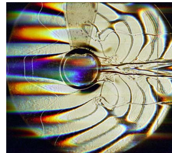
Внутренние волны и висящие разрывы в стратифицированном течении за цилиндром
