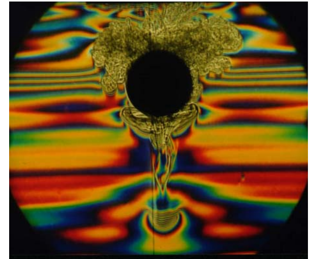
Автокумулятивная струя и внутренние волны, возникающая при свободных колебаниях сферы на горизонте нейтральной плавучести в непрерывно стратифицированной жидкости
